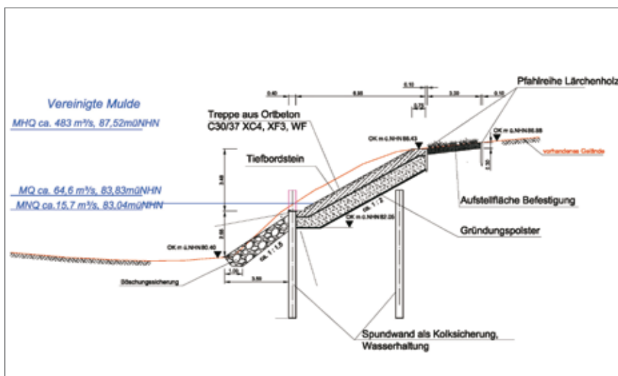
Bild 6: Regelquerschnitt Treppenanleger
