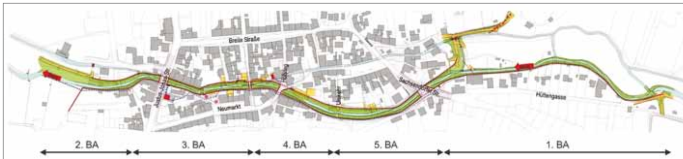
Bild 9: Übersichtslageplan Hochwasserschutz Eisfeld, (Quelle: HSP)
